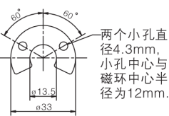
开口磁环垫片
